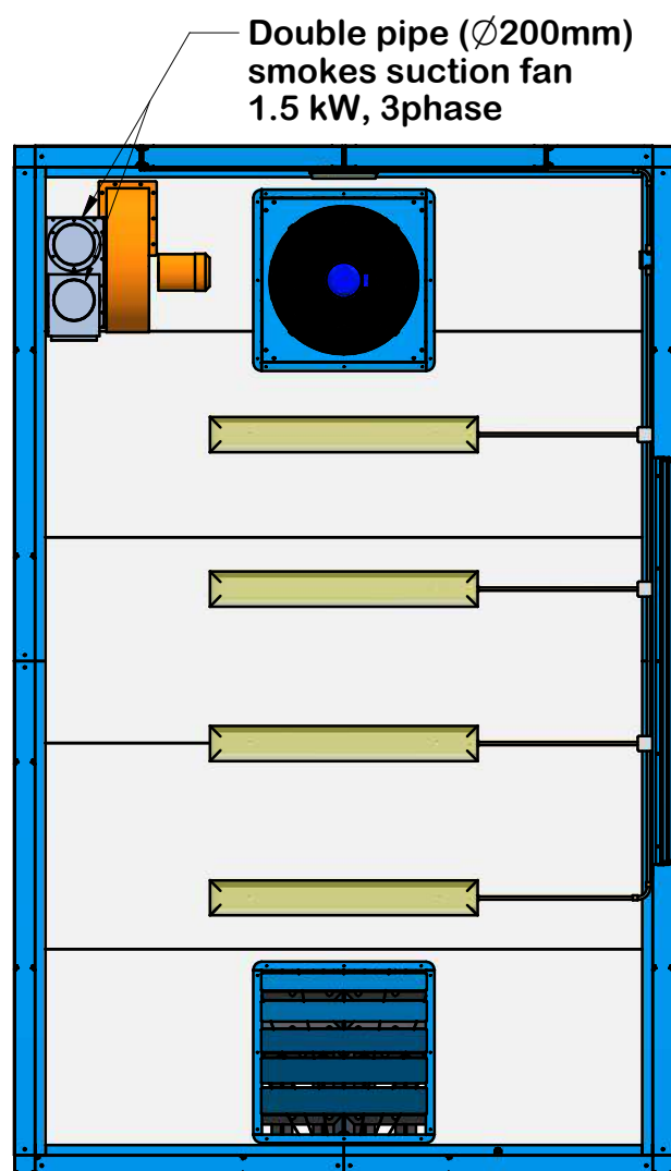
B-B
