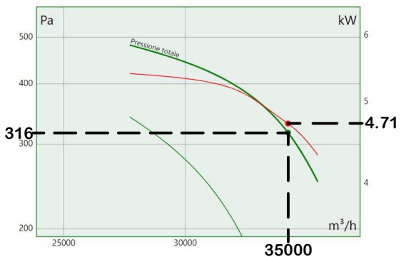
F Grafico riferito ad aria a 20 °C - altitudine 0 m - \rho = 1.204 \text{ kg/m}^3
